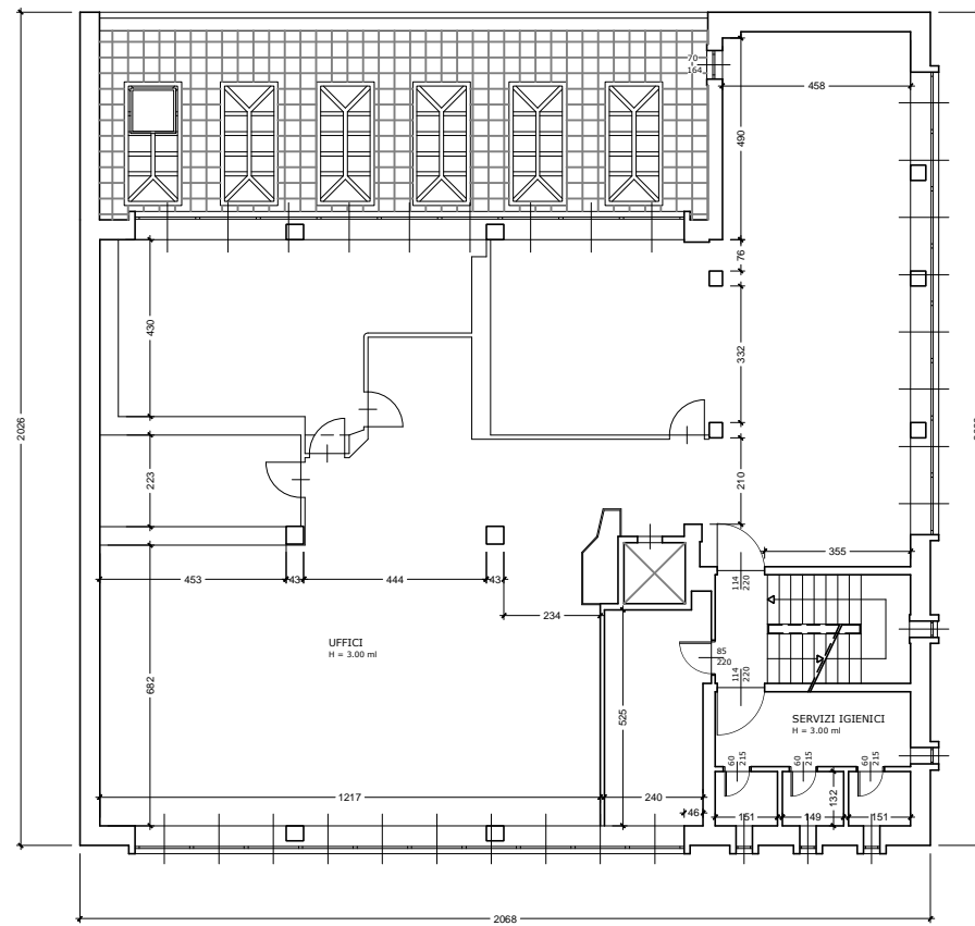
PIANO PRIMO - VIA GIUSTINIANI, 20 - RECCO - GE
