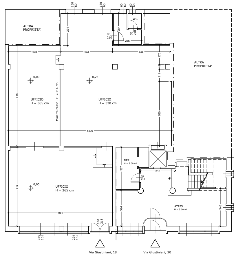
PIANO TERRA - VIA GIUSTINIANI, 18 e 20 - RECCO - GE
