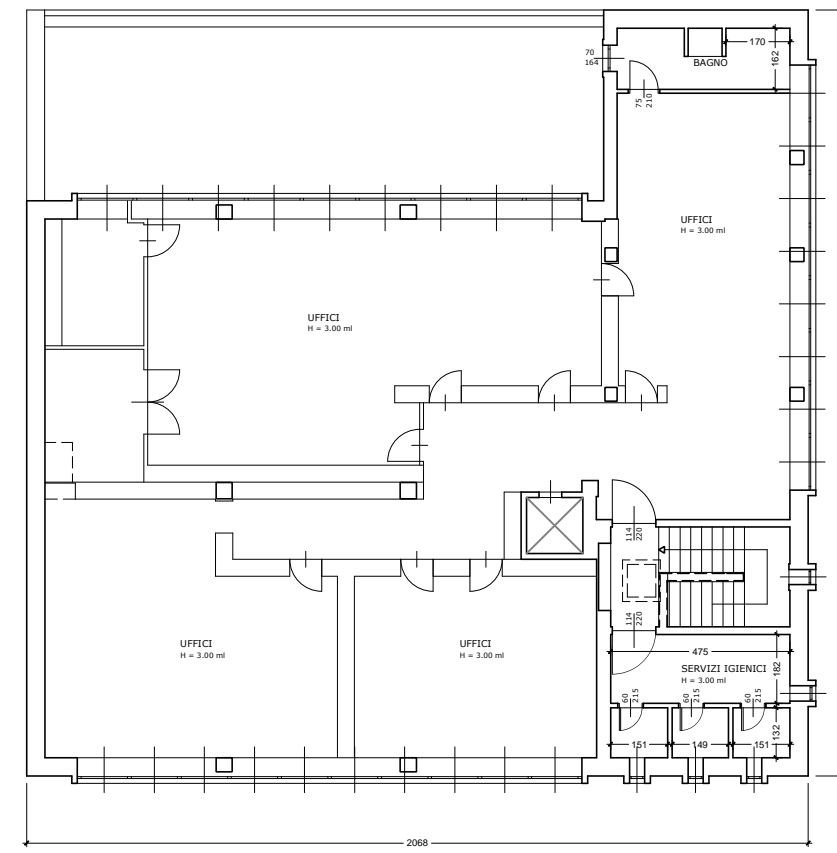
PIANO SECONDO - VIA GIUSTINIANI, 20 - RECCO - GE
